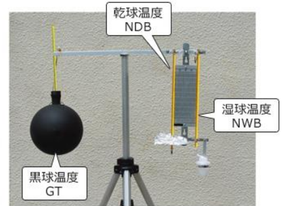
暑さ指数(WBGT)測定装置
