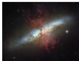
M82
