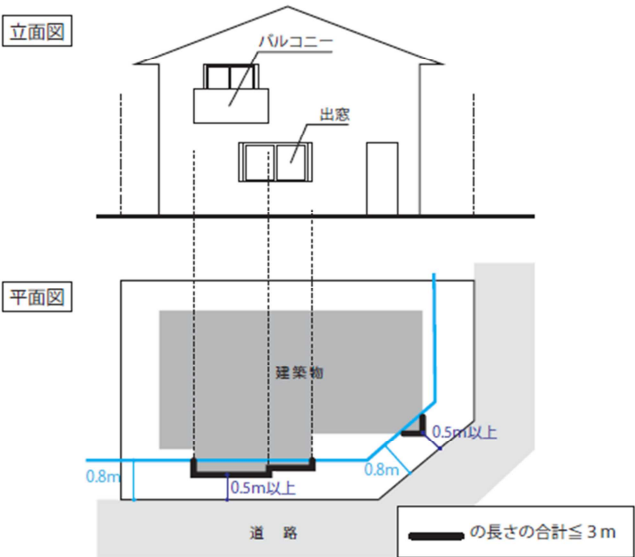
【図 2】 建築壁面の位置の制限（緩和規定）
