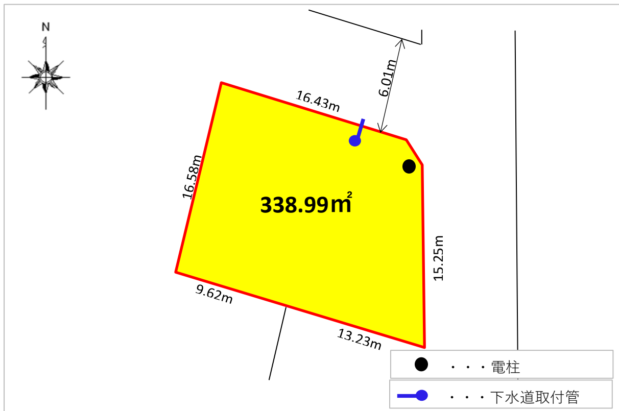
明細図
