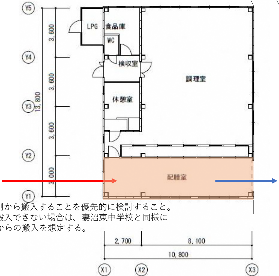
1階平面図 S=1/200
